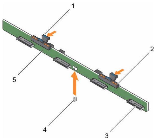
Ilustración 60. Extracción e instalación del plano posterior de la unidad de disco duro (x4) de 3,5 pulgadas
