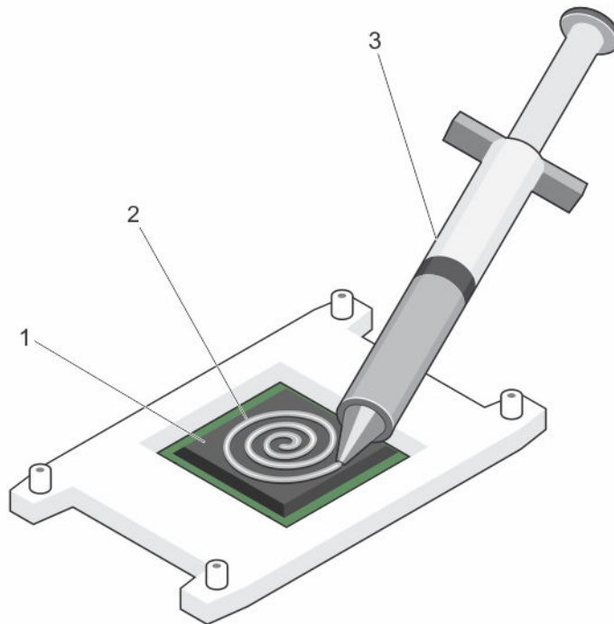
Ilustración 26. Aplicación de la grasa térmica en la parte superior del procesador
