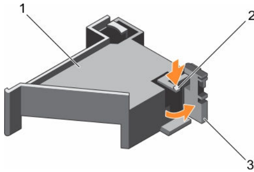
Ilustración 28. Apertura y cierre del pestillo del soporte de tarjeta PCIe
