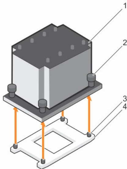
Ilustración 21. Extracción e instalación de un procesador
