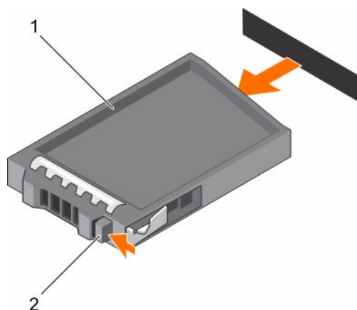
Ilustración 49. Extracción e instalación de una unidad de disco duro de relleno de 2,5 pulgadas
