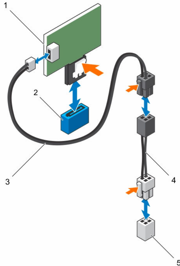
Ilustración 20. Extracción e instalación de SATADOM
