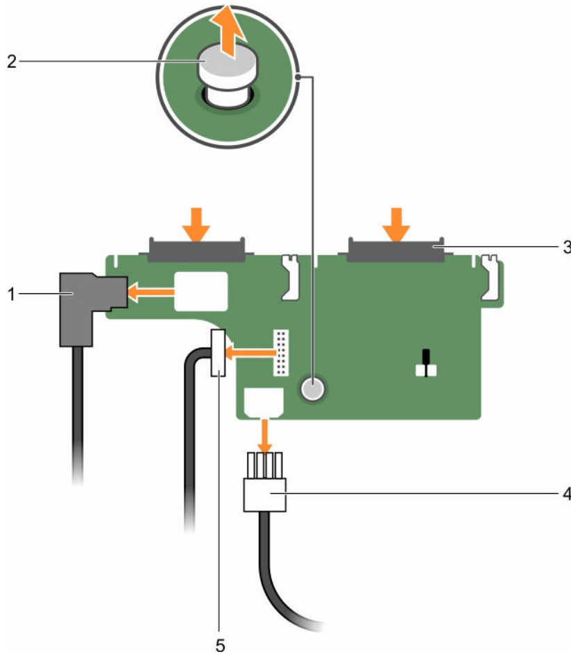
Ilustración 57. Extracción e instalación del plano posterior de la unidad de disco duro (x2) opcional de 2,5 pulgadas
