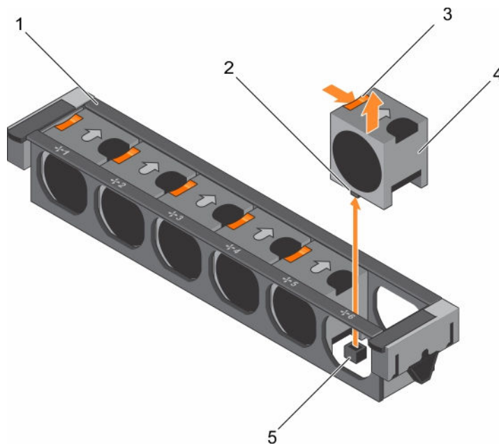
Ilustración 14. Extracción e instalación de un ventilador de refrigeración
