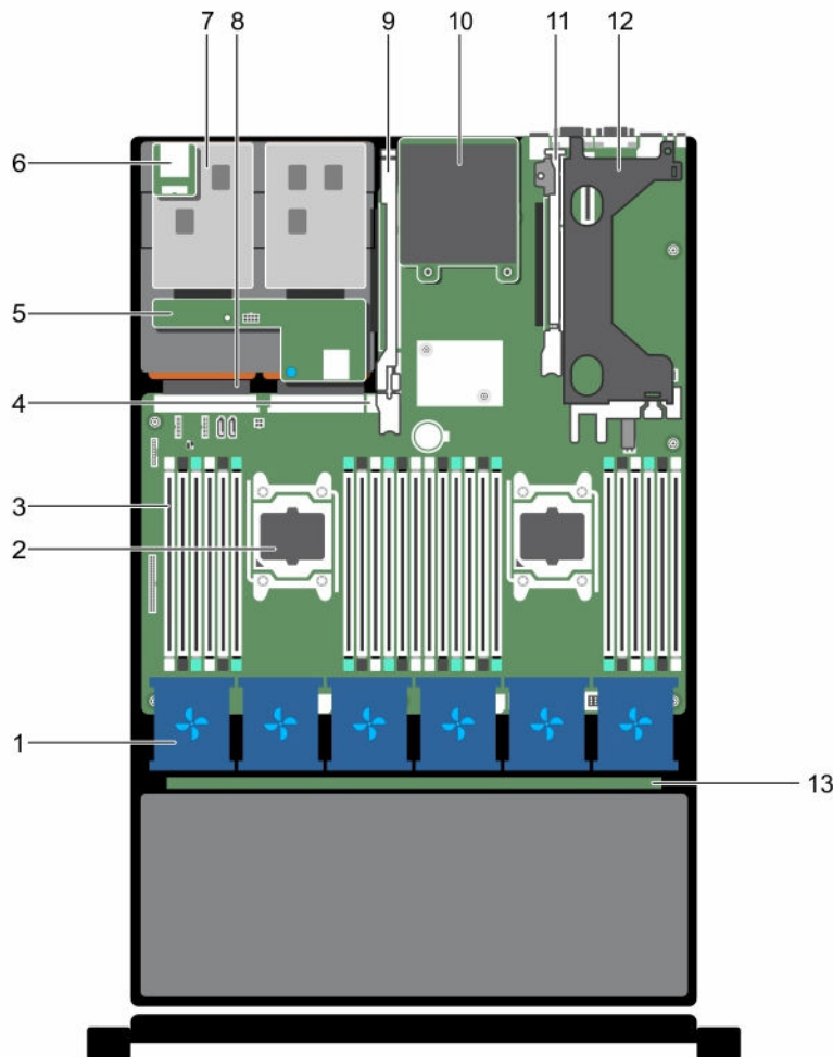
Ilustración 12. Interior del sistema: Dell XC730xd
