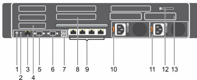
Ilustración 6. Características e indicadores del panel posterior
