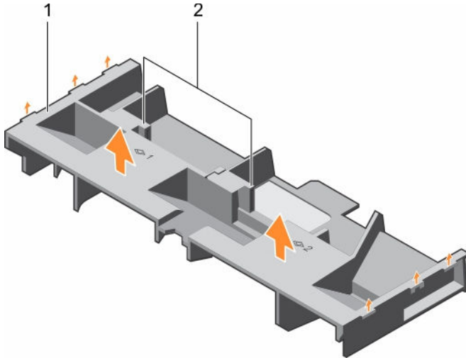
Ilustración 13. Extracción e instalación de la cubierta de refrigeración
