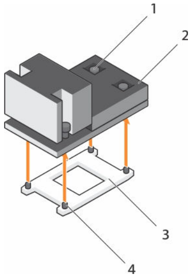
Ilustración 22. Extracción e instalación del disipador de calor del procesador
