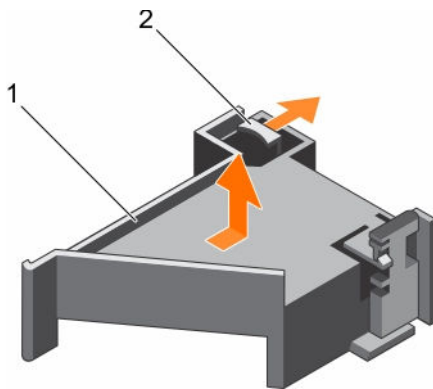
Ilustración 27. Extracción e instalación del soporte de tarjeta PCIe
