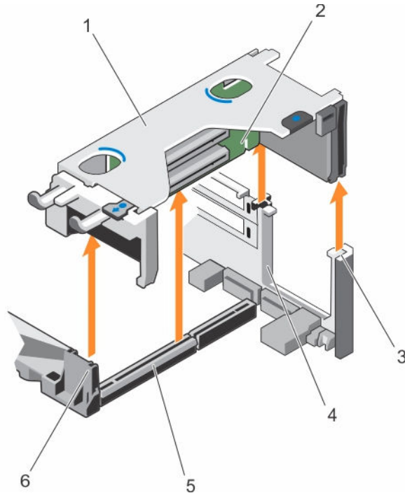
Ilustración 33. Extracción e instalación del soporte vertical 1 para tarjetas de expansión
