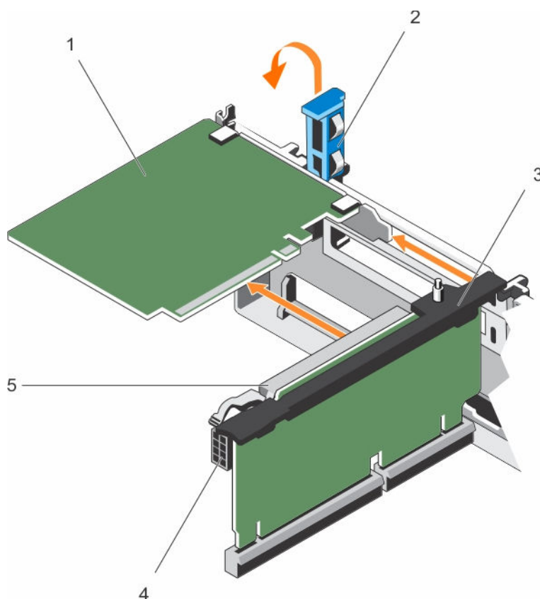
Ilustración 31. Extracción e instalación de una tarjeta de expansión de la tarjeta vertical de expansión 2 o 3
