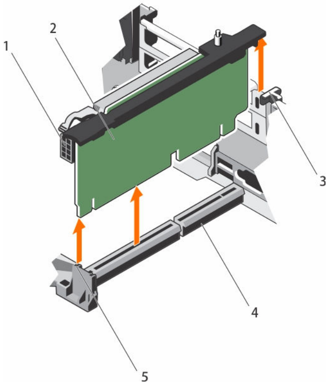
Ilustración 35. Extracción e instalación del soporte vertical 2 para tarjetas de expansión
