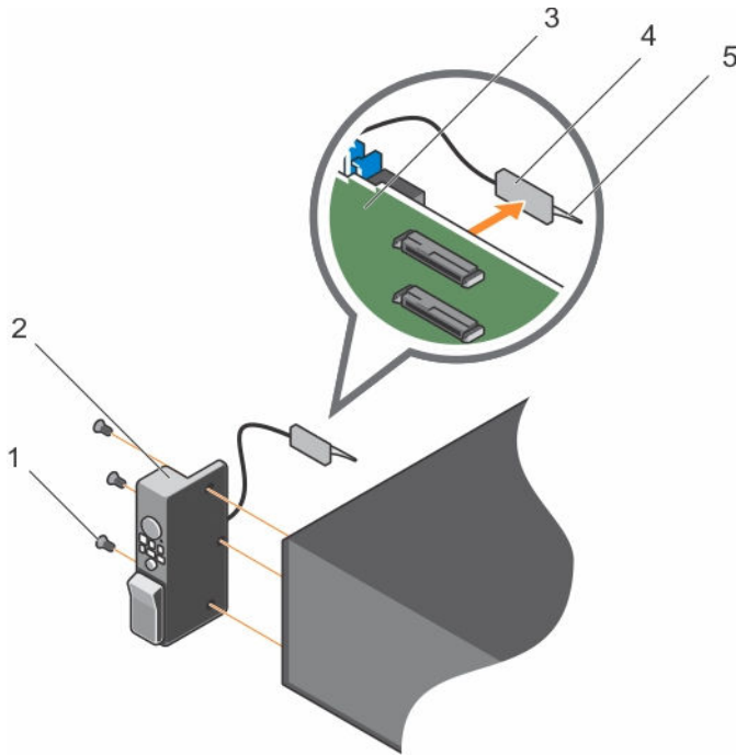
Ilustración 58. Extracción e instalación del panel de control
