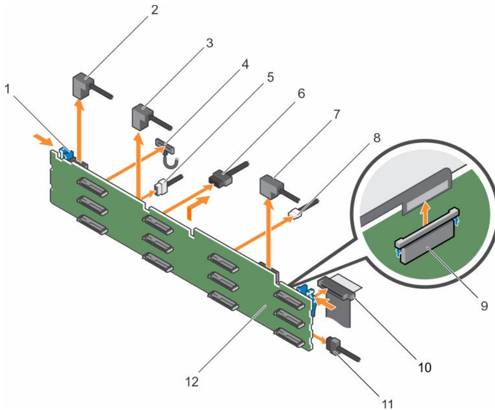
Ilustración 56. Extracción e instalación del plano posterior SAS/SATA (x12) de 3,5 pulgadas
