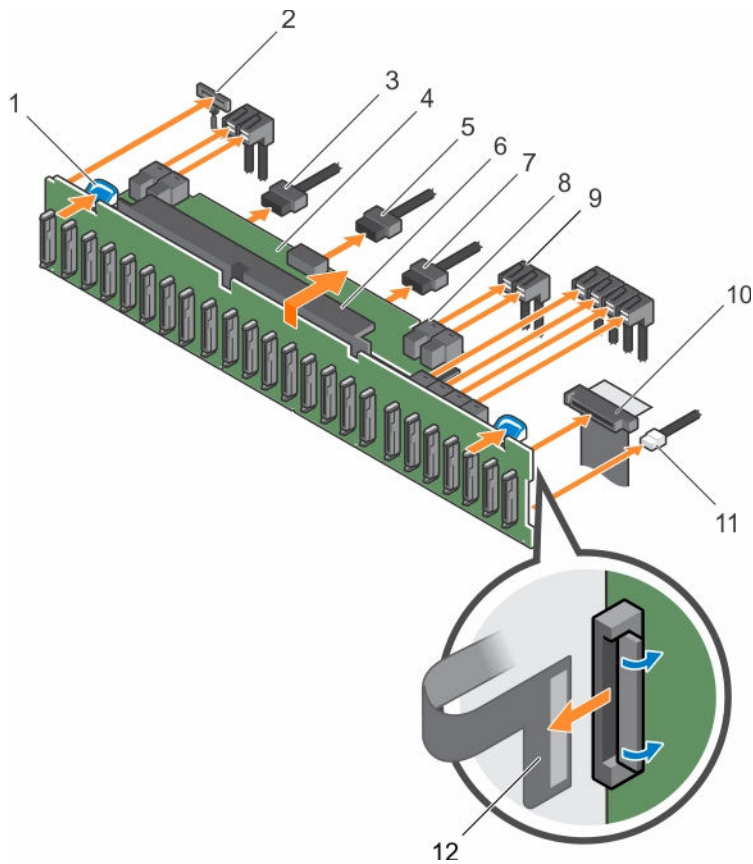
Ilustración 54. Extracción e instalación del plano posterior SAS/SATA (x24) de 2,5 pulgadas
