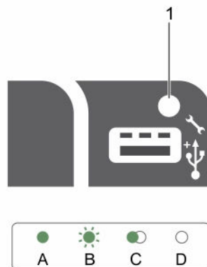
Ilustración 5. Indicador LED de iDRAC directo
