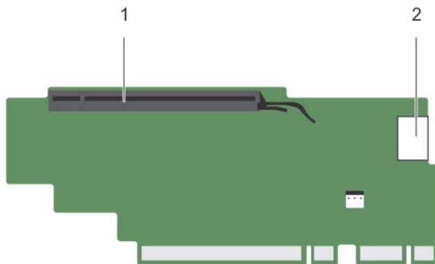
Ilustración 39. Identificación de los conectores del soporte vertical 3 para tarjetas de expansión (alternativo)
