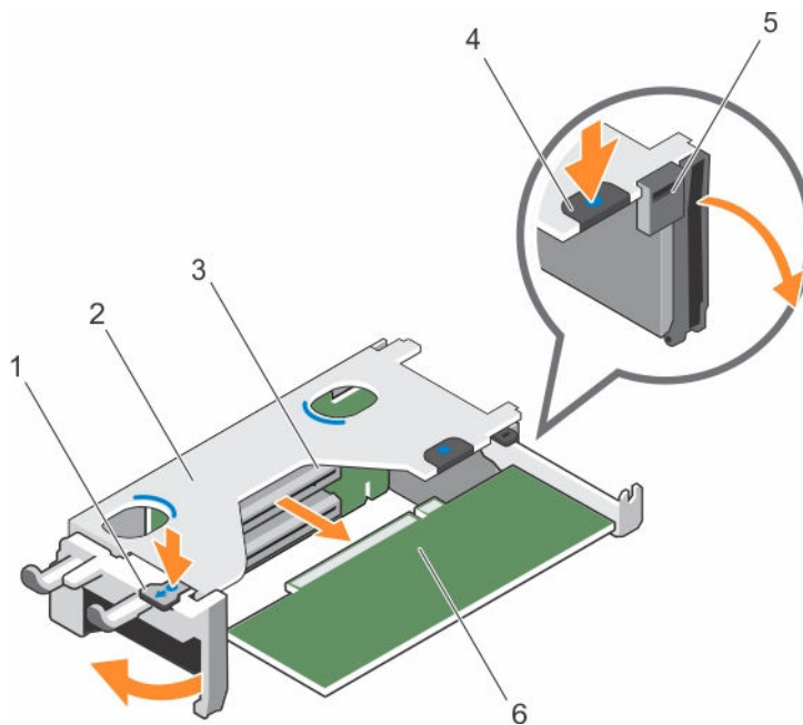
Ilustración 32. Extracción e instalación de la tarjeta de expansión del soporte vertical 1 para tarjetas de expansión
