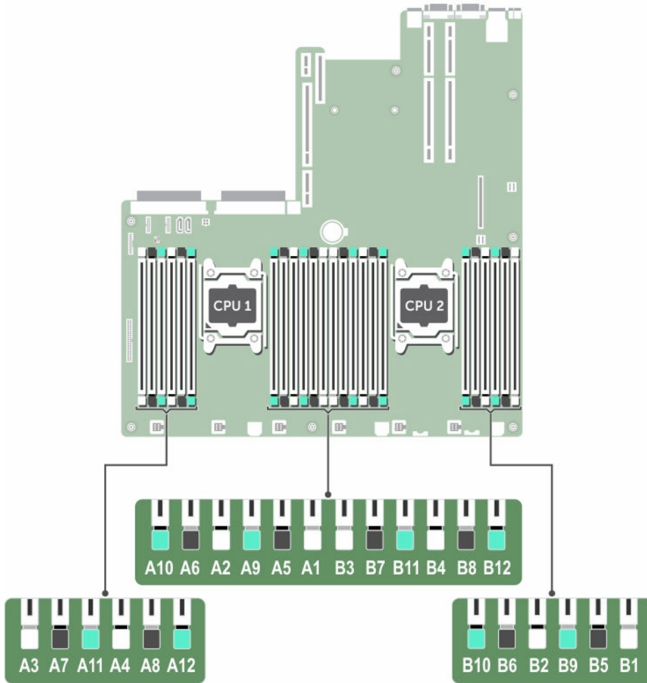
Ilustración 16. Ubicaciones de los zócalos de memoria
