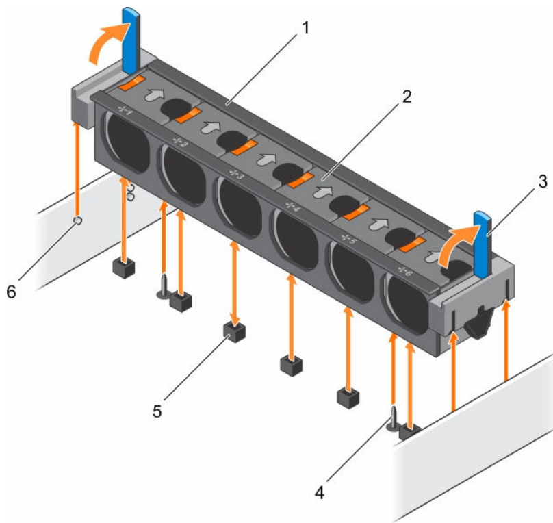
Ilustración 15. Extracción e instalación del ensamblaje del ventilador de refrigeración
