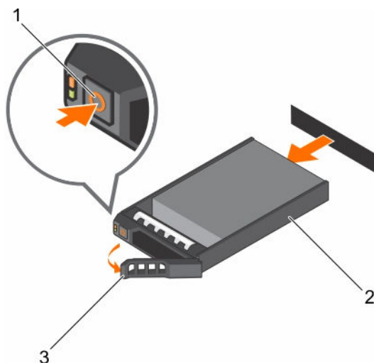
Ilustración 52. Extracción e instalación de una unidad de disco duro de intercambio directo
