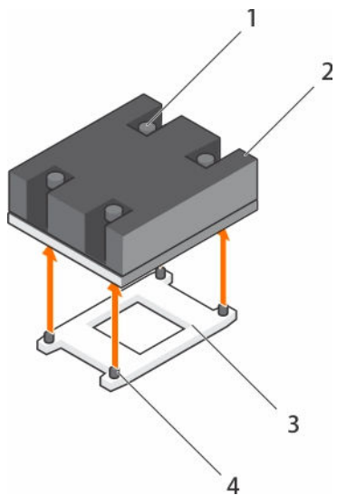
Ilustración 23. Extracción e instalación del disipador de calor del procesador
